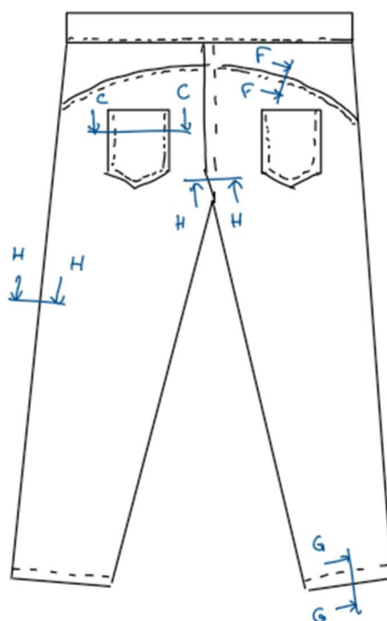
Coupe F-F
